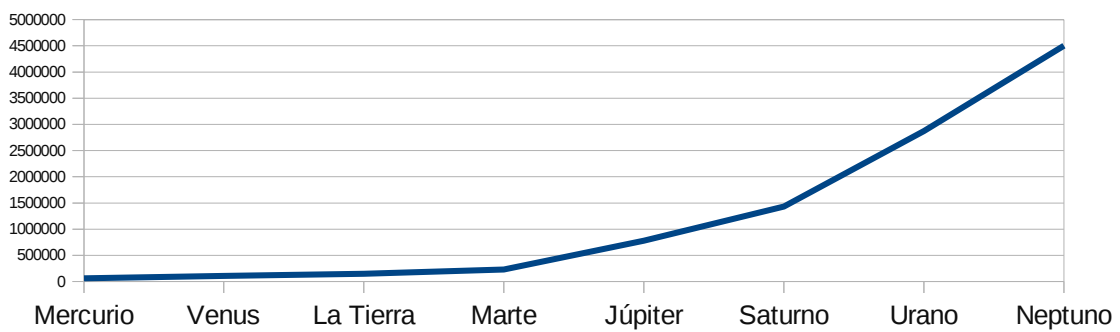
Distancia al Sol
